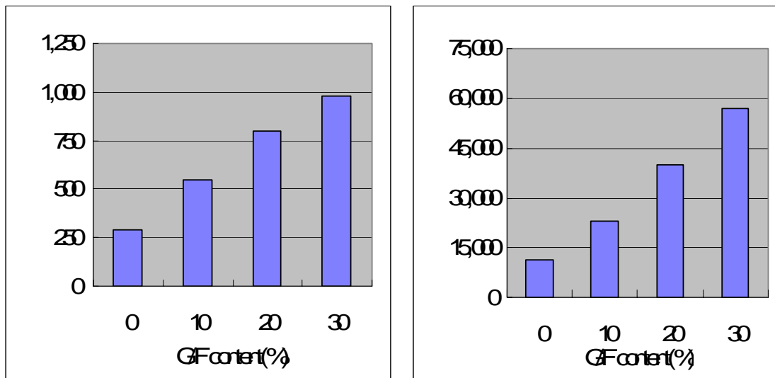
[图1 随着玻璃纤维钢化的物性保钢性效果]
